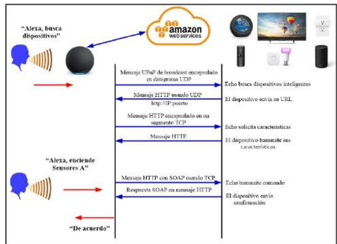
Figura 2. Comunicación entre el asistente Alexa y el ESP32-WROOM
